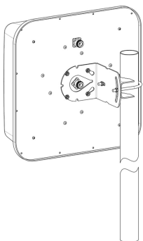
Рисунок 2 – Монтаж антенны
